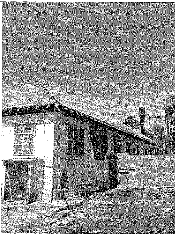
FOTO GERAL - DURANTE A SUBSTITUIÇÃO DO TELHAMENTO
